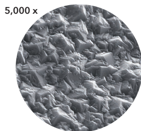
NexxZr Tool D 車針 表面均勻的鋒利鑽石晶體
