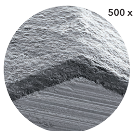
電子顯微鏡截面圖 顯示均勻一致, 約5微米的薄 鑽石塗層
