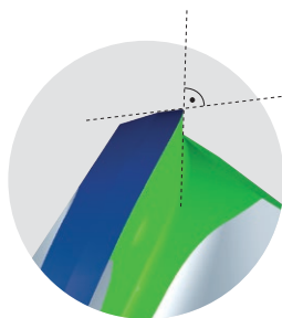
切削刀微觀幾何圖形的 CAD 示意圖
