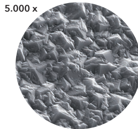
NexxZr Tool D glodalo Ujednačen izgled dijamantnih kristala s oštrim rubom
