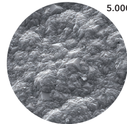
Konvencionalno glodalo Nepravilan izgled dijamantnih kristala s oštrim rubom
