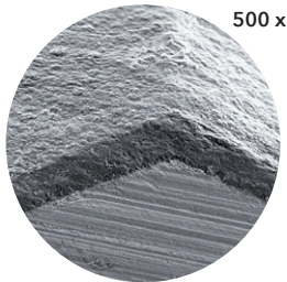
Slika SEM presjeka ujednačenog, pribl. 5 µm tankog dijamantnog premaza
