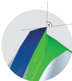
CAD prikaz mikrogeometrije reznog ruba
